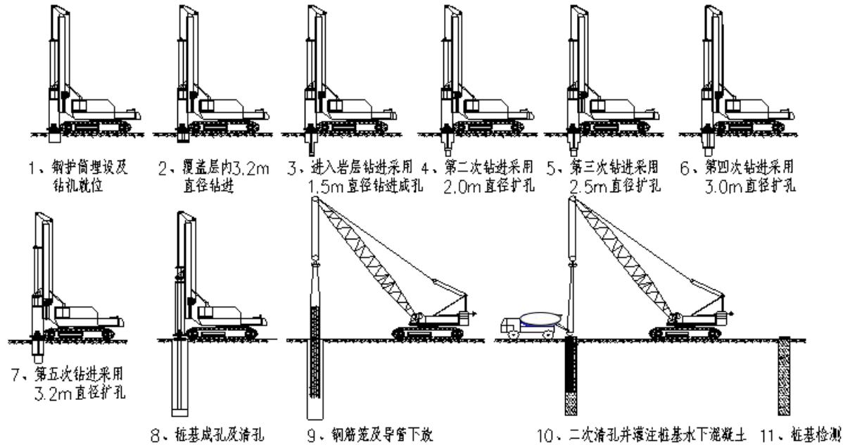
图 1 “分级成孔”施工示意图
