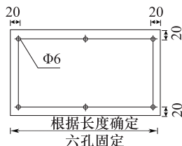
图 3-2 六孔固定安装示意图
