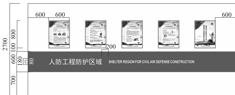
图 8-3 宣传标牌安装示意图
