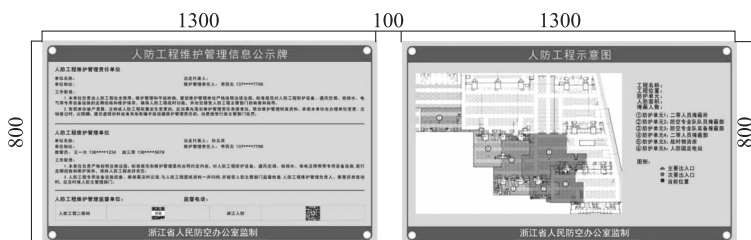
图4-1 人防工程示意图、人防工程维护管理信息公示牌安装示意
