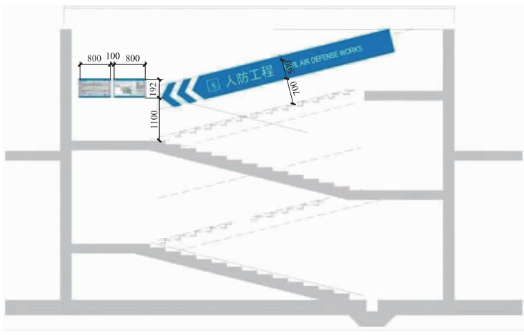
图 5-5 自行车坡道两侧墙面标识示意
