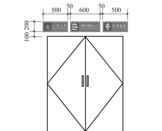
图 6-2 人防功能标牌安装示意图二
