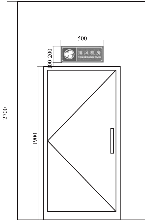
图 6-1 人防功能标牌安装示意图一
