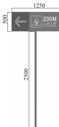
图 5-1 户外导引标牌安装示意
