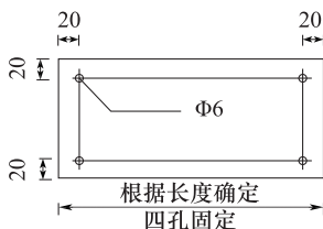
图 3-1 四孔固定安装示意图
